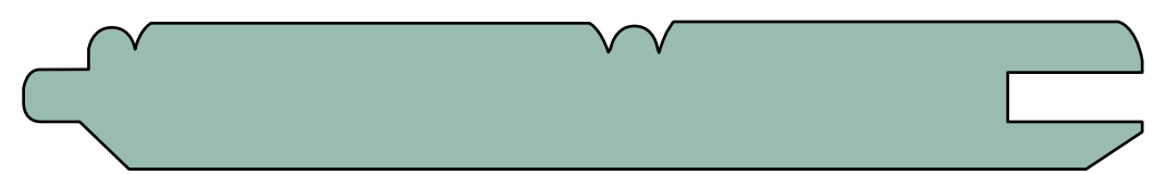
1 X 6 "C & BTR" EDGE & CENTERBEAD / V-JOINT
